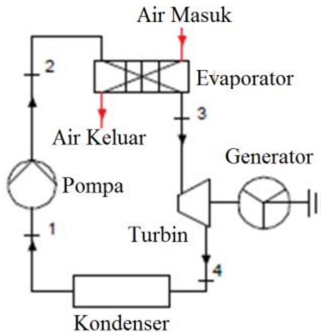
Gambar 1. Komponen-komponen utama sistem ORC [6]
