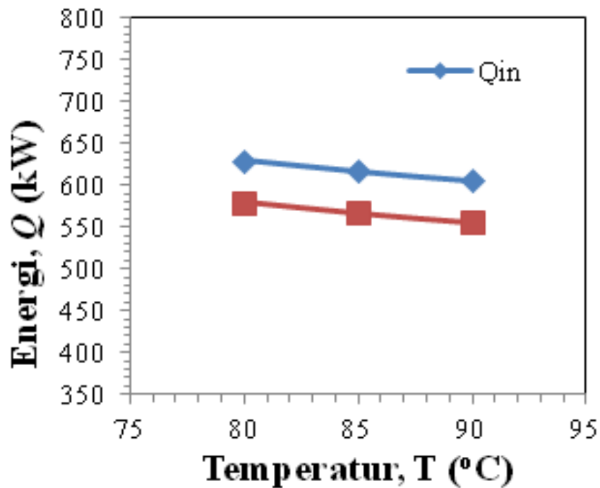
Gambar 7. Perbandingan Q_{in} dan Q_{out}
