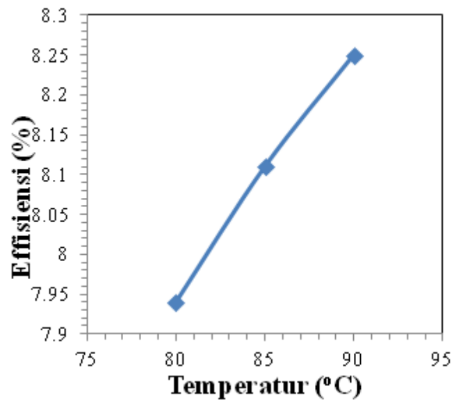
Gambar 9. Efisiensi sistem ORC
