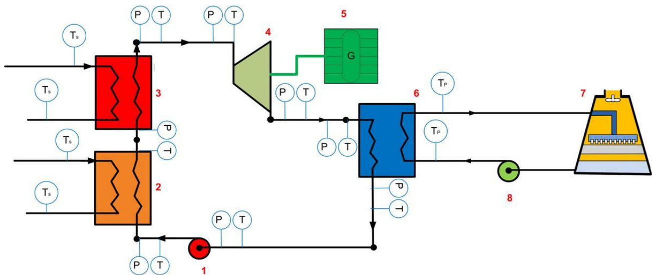
Gambar 5. Schematik ORC untuk penerapan Eksperimen
