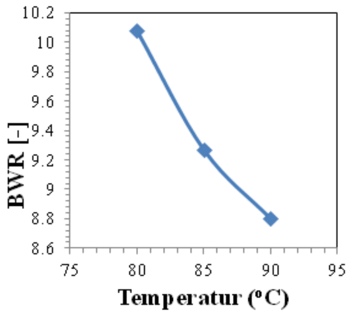
Gambar 8. Nilai BWR akibat variasi temperatur
