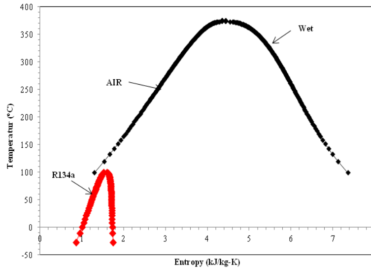
Gambar 6. Kurva T-S Diagram air dan R134a
